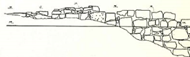
Mur de contenció, carrer del Pont (Balaguer, la Noguera). Escala 1:100.
